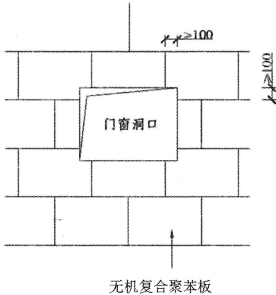
图 5.2.5 门窗口处无机复合聚苯板图
