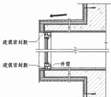
图 A.0.5 凸窗保温构造
