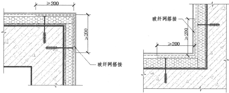
图 A.0.1 阴、阳角部位保温构造
