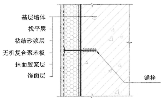
图 5.2.1 系统构造图
